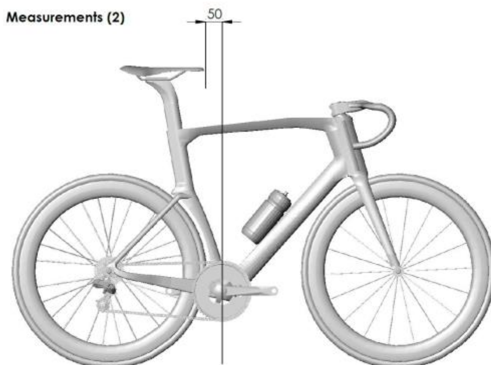
rysunek „Wymiary (2)”
